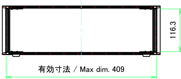
A-A ( 1 : 6 )
