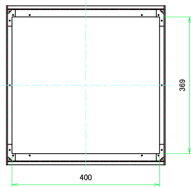
B-B ( 1 : 6 )
